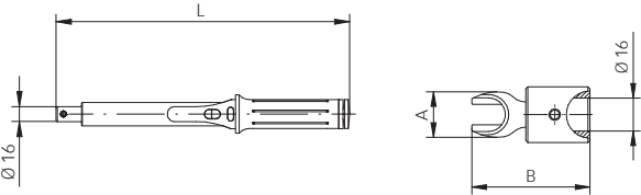
扭矩扳手
