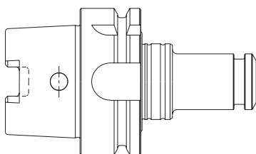
刀柄
