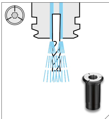
CF：集中式冷却
